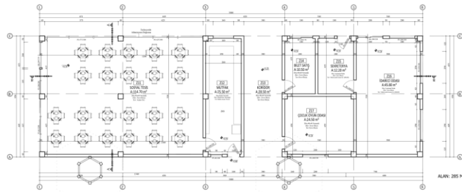
B BLOK ZEMİN KAT PLANI Ö:1/50
