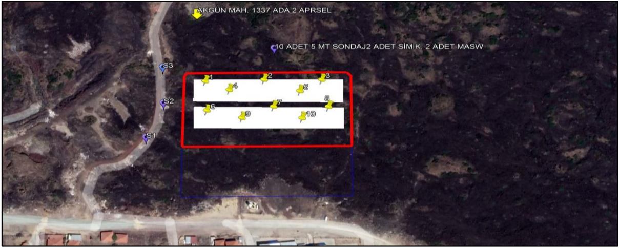
Tekstil Atölyesi Sondaj Noktaları Vaziyet Planı
