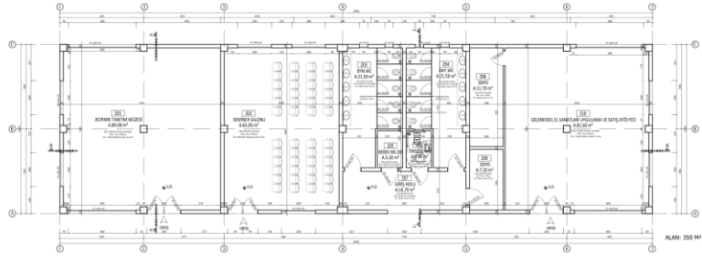
A BLOK ZEMİN KAT PLANI Ö:1/50
